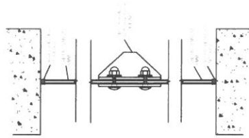
SECCION A-A
